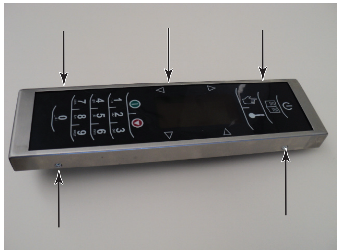
Remove 5 Escutcheon Screws
